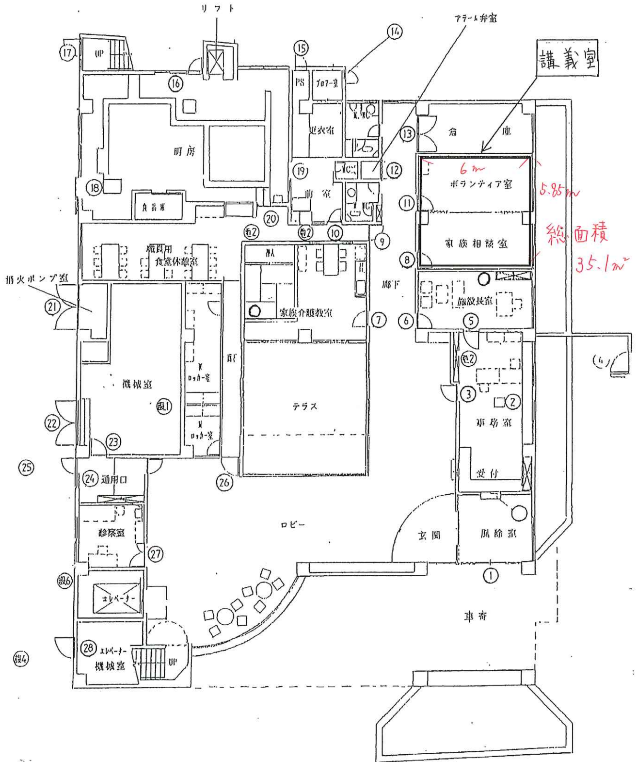
1階平面図
